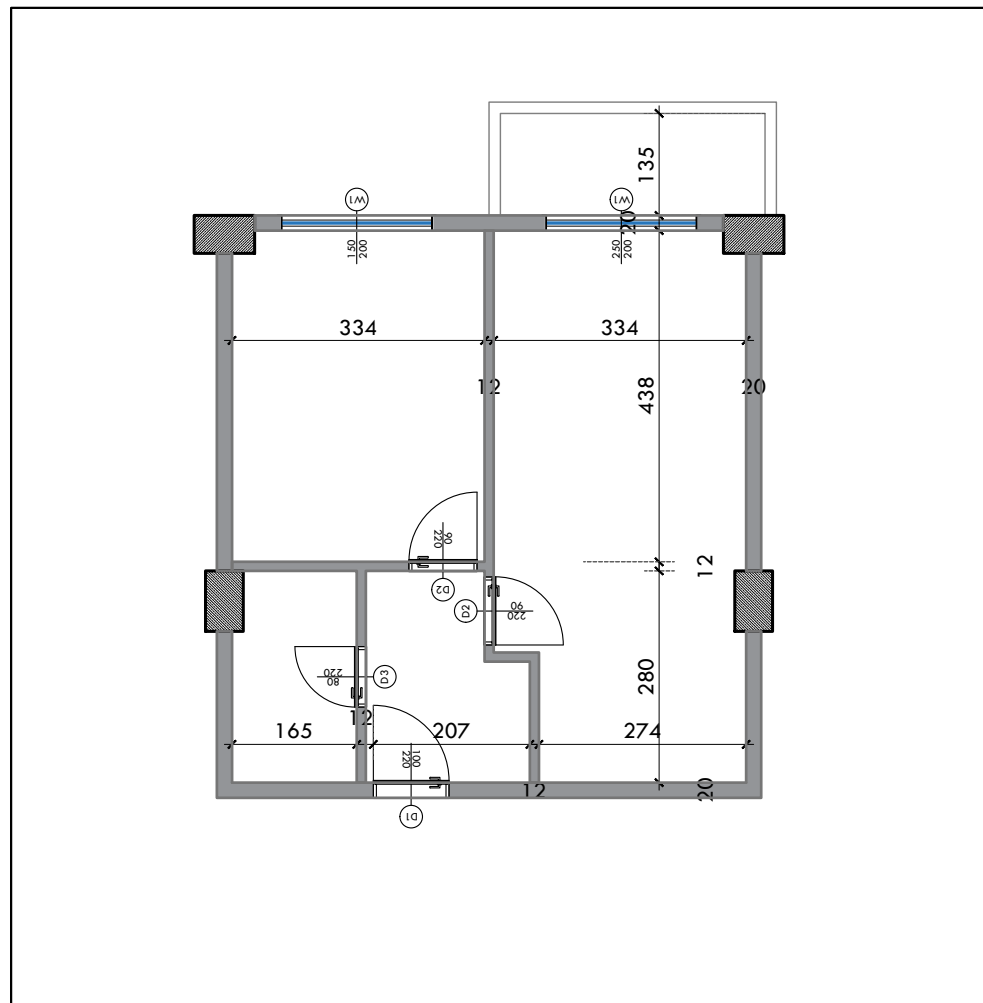
PLANIMETRIA E APARTAMENTIT - PERMASIM SHKALLA 1:100
