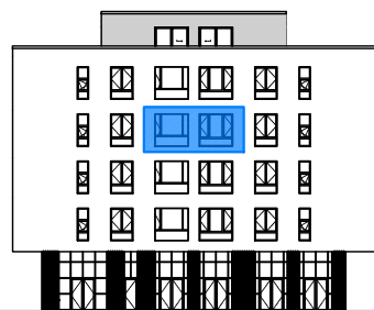
POZICIONI I APARTAMENTIT NE ALTIMETRI - FASADA VERIORE
